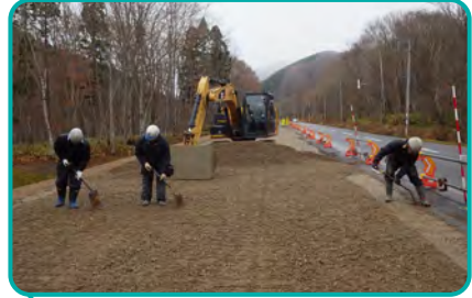
● 舗装工 舗装作業前 下層路盤敷均し
